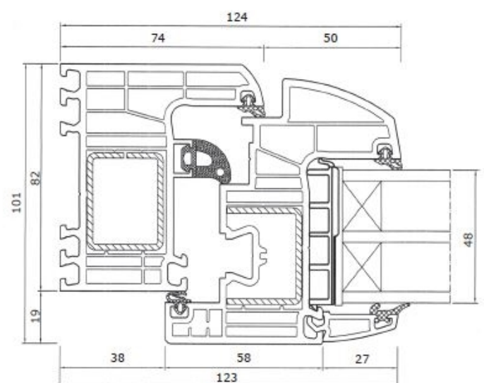
Euro 7000, halbfächenversetzt mit 74 mm Blendrahmen
