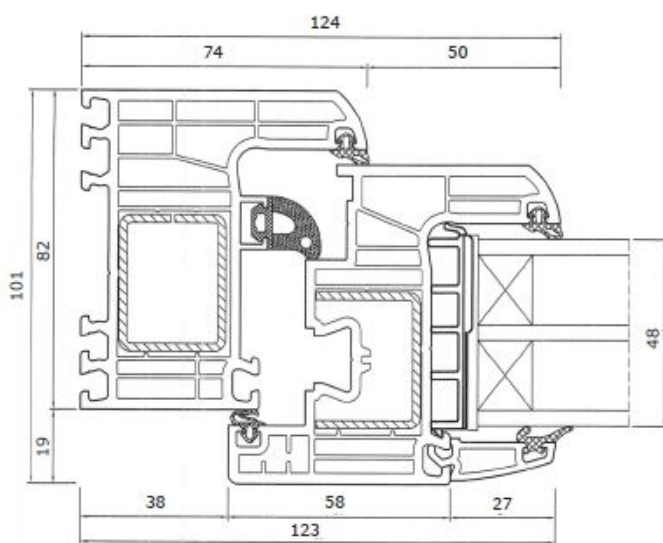
Euro 7000, flächenversetzt, classic mit 74 mm Blendrahmen
